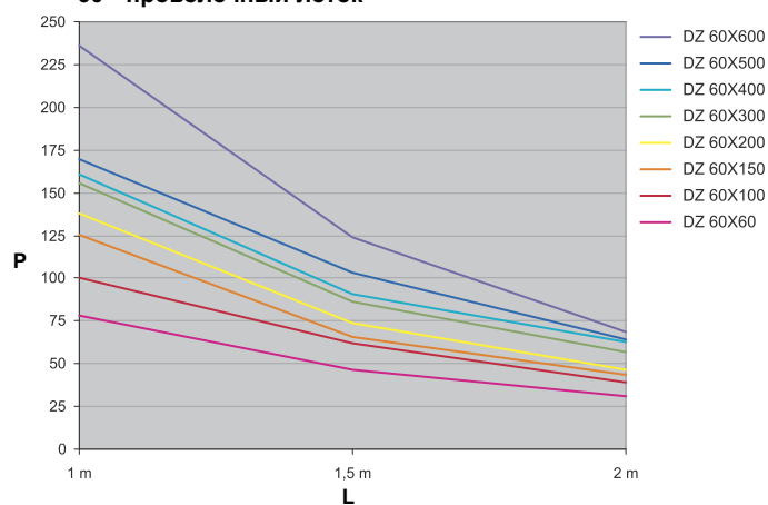
60 - проволочный лоток
