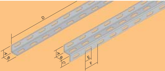
Л и Z профиль
