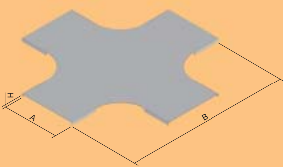
крышка ответвителя крестообразного
