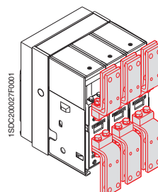
Выводы для подключения спереди
