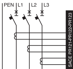
Трехполюсные автоматические выключатели
