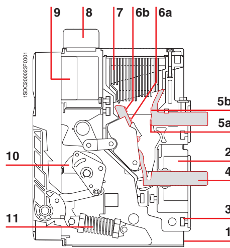
Селективный автоматический выключатель E1 B-N, E2 B-N-H, E3 N-S-H-V, E4 S-H-V, E6 H-V
