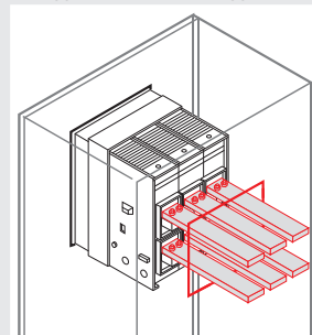
Горизонтальные выводы с подключением сзади
