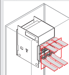
Плоские выводы с подключением сзади
