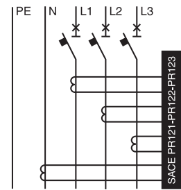
Трехполюсные автомат. выключатели с внешней нейтралью
