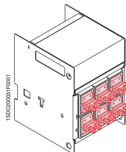
Плоские выводы
