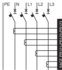
Четырехполюсные автомат. выключатели
