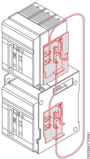
вертикальная взаимная блокировка
