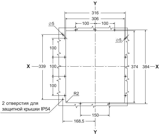
Отверстия в двери отделения
