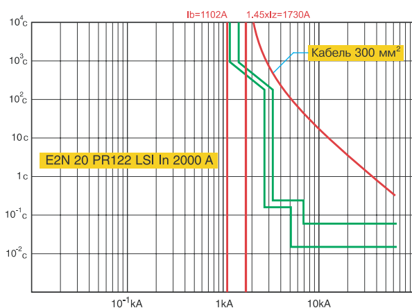
Кривая "время - ток" LLL
