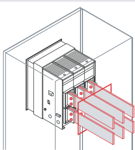
Вертикальные выводы с подключением сзади
