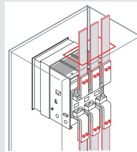
Выводы с подключением спереди
