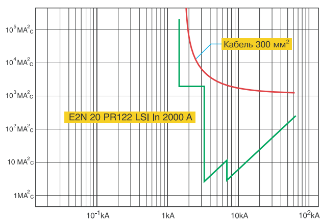
Кривая удельной энергии рассеивания LLL
