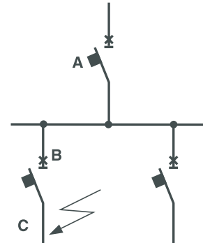
Электрическая схема с селективным согласованием устройств защиты.
