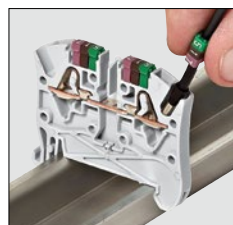
Безыструментальный монтаж жесткого проводника и гибкого с наконечником в клеммы с шагом до 6 мм
