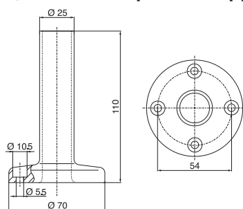
Цоколь со встроенной трубкой
