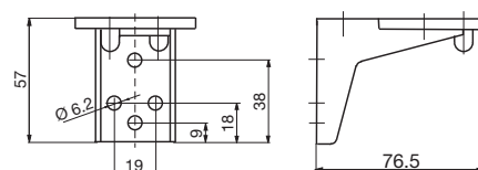
Кронштейн для монтажа на поверхности
