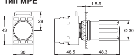
Кнопка аварийной остановки, тип МРЕ
