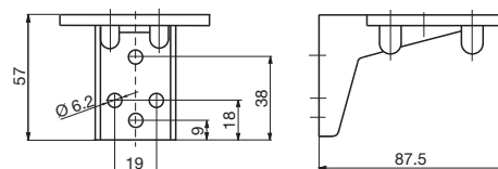
Кронштейн для монтажа на трубе
