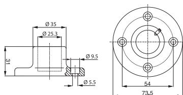
Цоколь для трубки, металл
