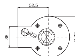
Кронштейн для монтажа на поверхности
