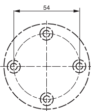
Схема сверления отверстий для сигнальных стоек К 70
